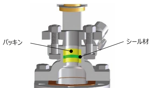
シール材を充填する空間がある場合
