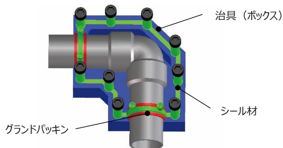
シール材を充填する空間がない場合
